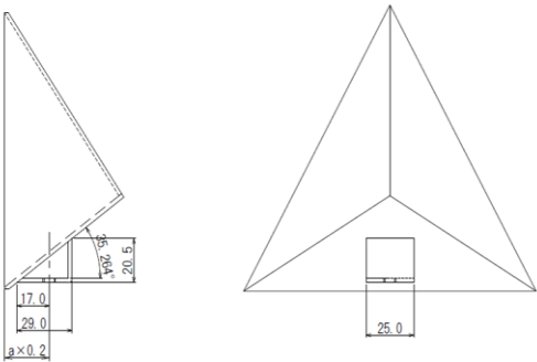
取付部説明図 a=0.078~0.139m例
